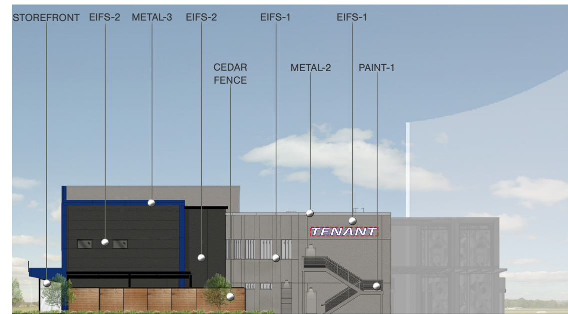
Right Elevation
